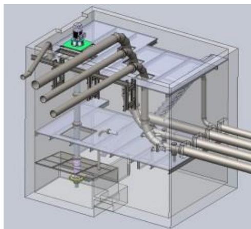
Příklad potrubního vedení
