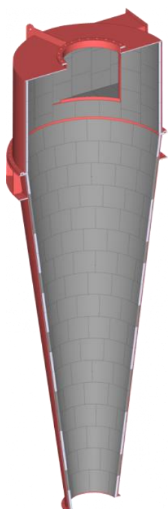
Vyložení cyklonu
