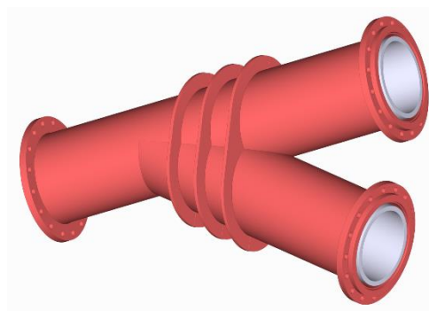
Odbočka s žebrovým vyztužením
